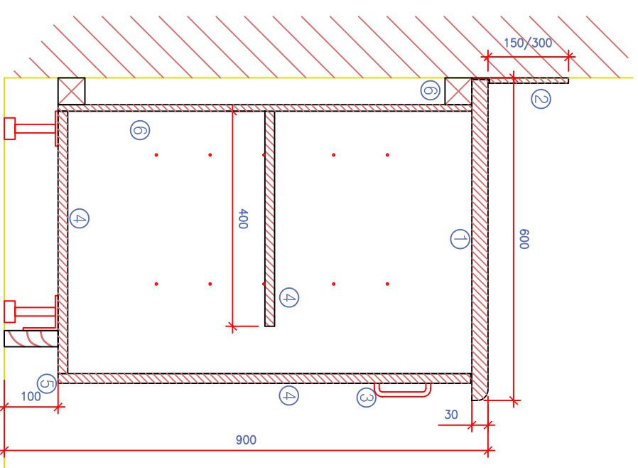
elevation b-b
