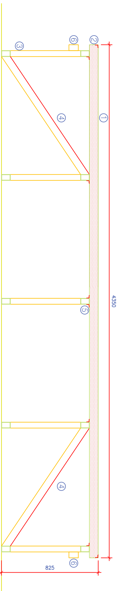
elevation b-b
